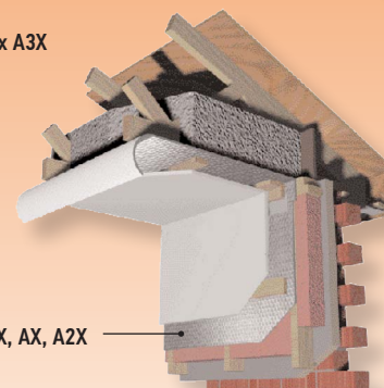
Reflex A3X, AX, A2X
